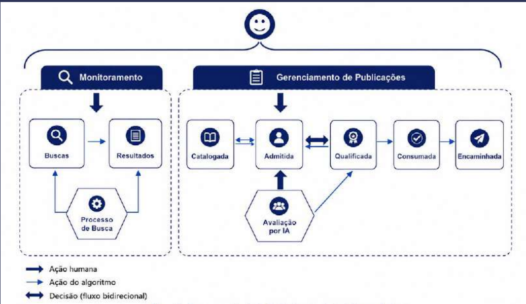
Figura 1. Fluxos operacionais do GualA. As setas cheias indicam ação humana.
